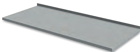
Pracovní deska se zadním lemem - výška 40 mm, zadní lem - 40 mm
