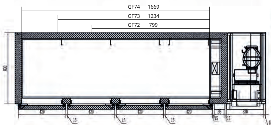
Púdorys
